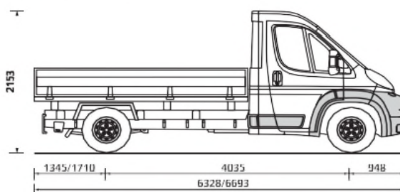
Ploščad z enojno kabino L3/L4
