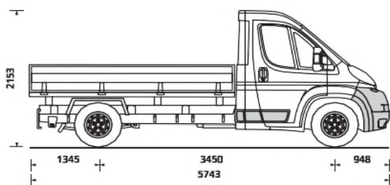
Ploščad z enojno kabino L2
