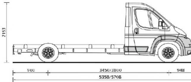
Šasija s kabino L2/L2S
