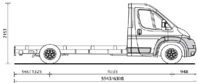
Šasija s podaljšano kabino L3/L4
