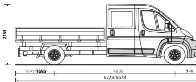
Ploščad s podaljšano kabino L3/L4
