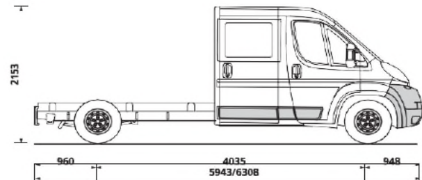
Šasija s podaljšano kabino L3/L4
